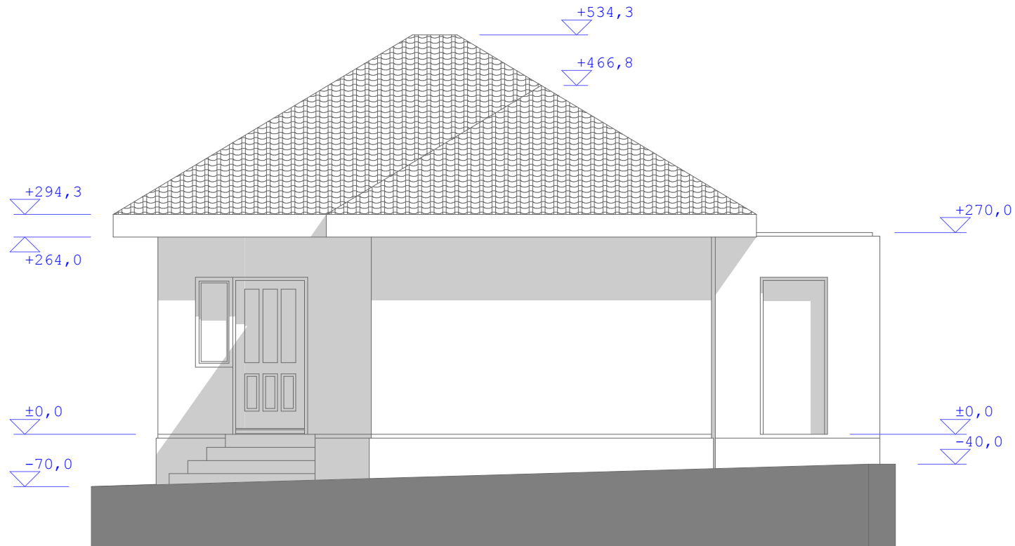
FAȚADA NORD-EST - SITUAȚIA EXISTENTĂ 1:70
